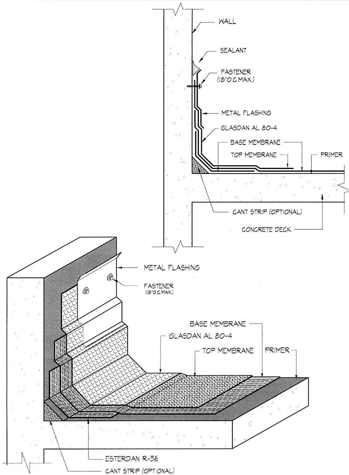
DETALLE #2
